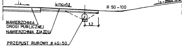
PRZEKRÓJ 1-1
